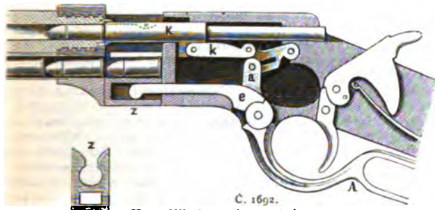
Henry-Winchestrovka se zámkem nataženým.
